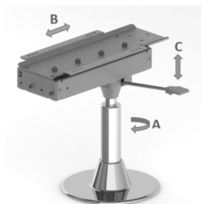
A: rotazione di 360° con auto-allineamento alla posizione di riposo B: traslazione di 180 mm con ritorno automatico alla posizione di riposo C (opzionale): regolazione in altezza di 50 mm con auto-allineamento alla posizione "tutto alto"
