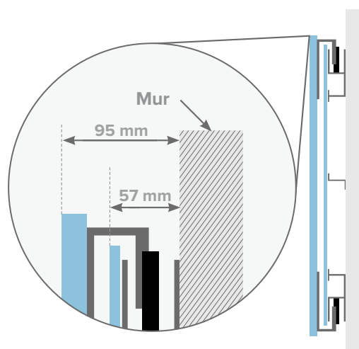
Vue latérale
